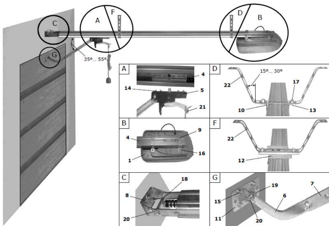
Рис. 2. Монтаж устройства
